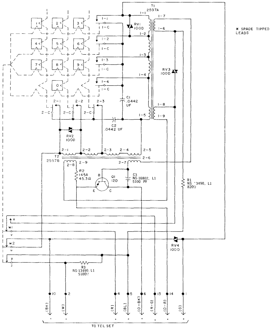
Fig. 8 -- 25E Dial
