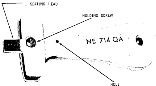
Fig. 1 - NE714QA Tool
