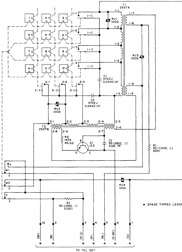
Fig. 4 - 35A3 Dial
