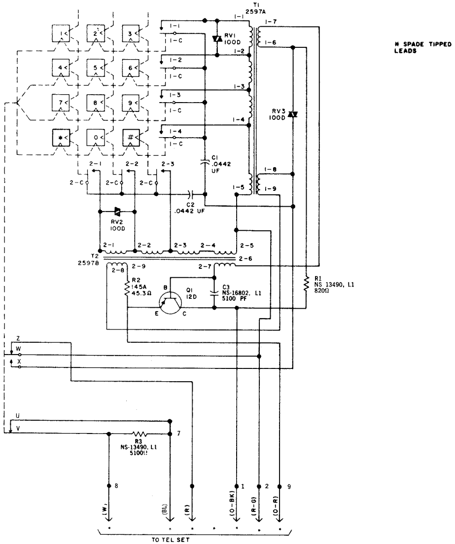
Fig. 6A - 35Q3E Dial
